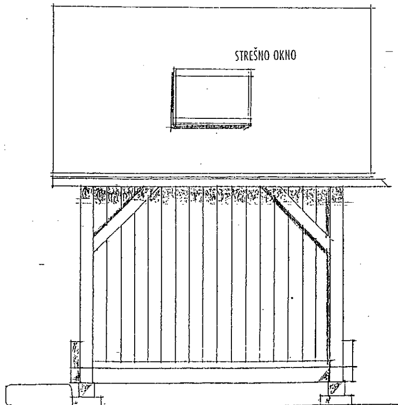
SEVERNA FASADA
