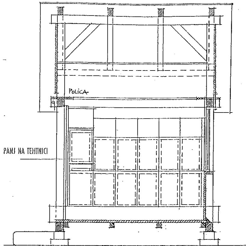
VZDOLŽNI PREREZ
